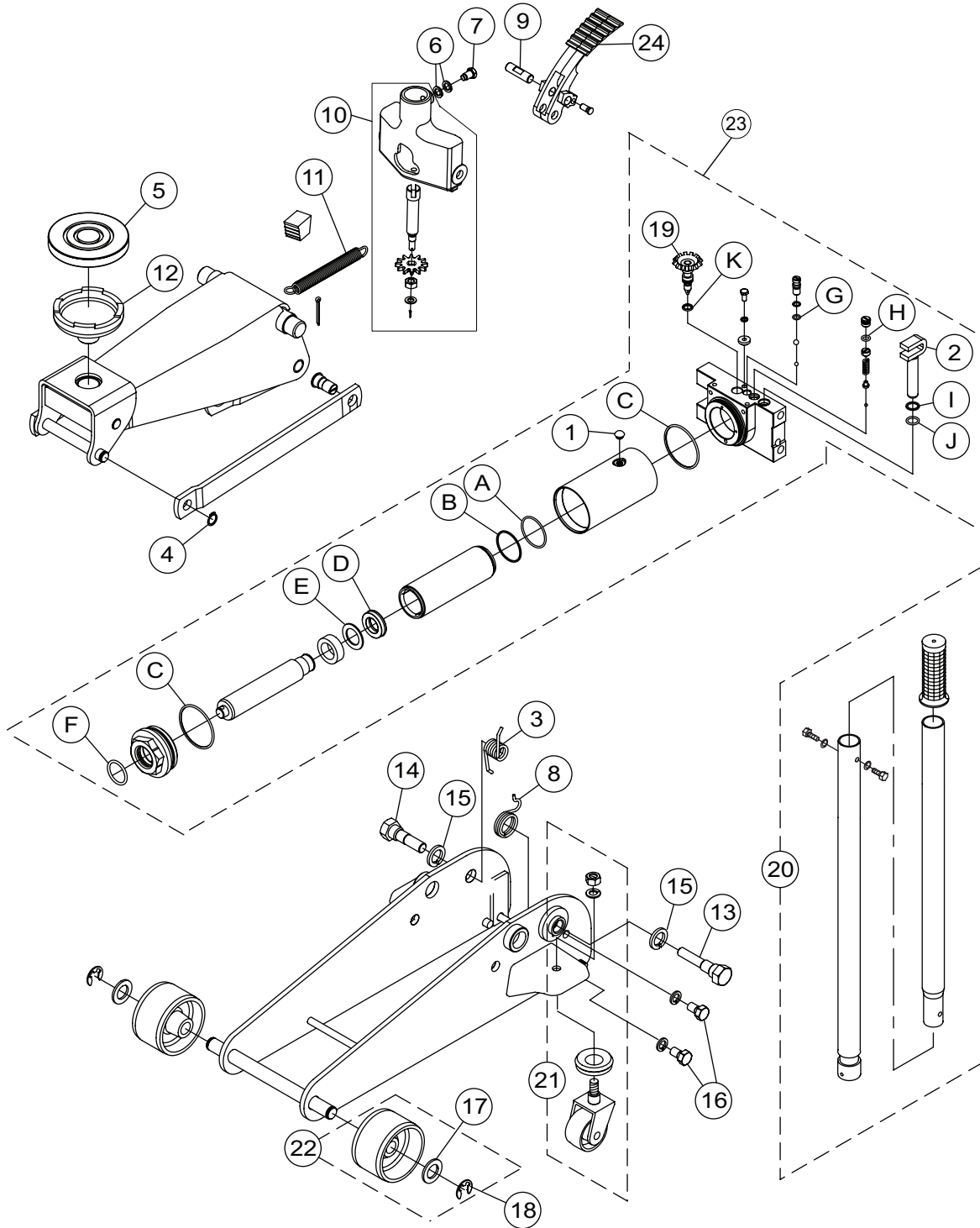
Figura 2: Ilustración de piezas de repuesto para el modelo BH6034B
