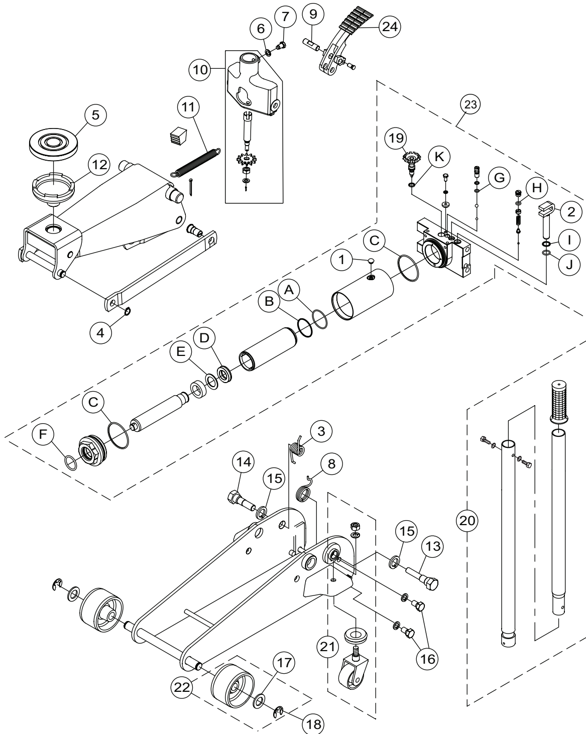
Figure 2 : Illustration des pièces de rechange du modèle BH6034B
