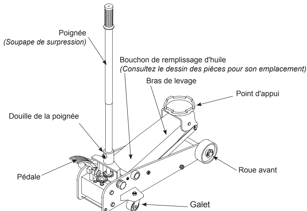
Figure 1 : Pièces d'un cric type
