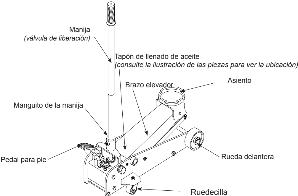
Figura 1: Nomenclatura habitual de un gato
