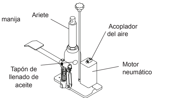
Figura 1: nomenclatura de los modelos T-5500/T-5501
